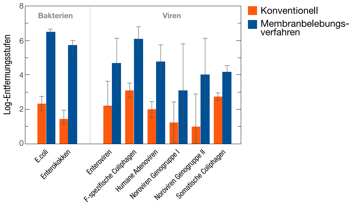
Abb. 2: Vergleich von konventionellen Belebungsverfahren und Membranbelebungsverfahren bezüglich der Entfernung typischer Bakterien und Viren (zusammengestellte Literaturdaten aus [6])
